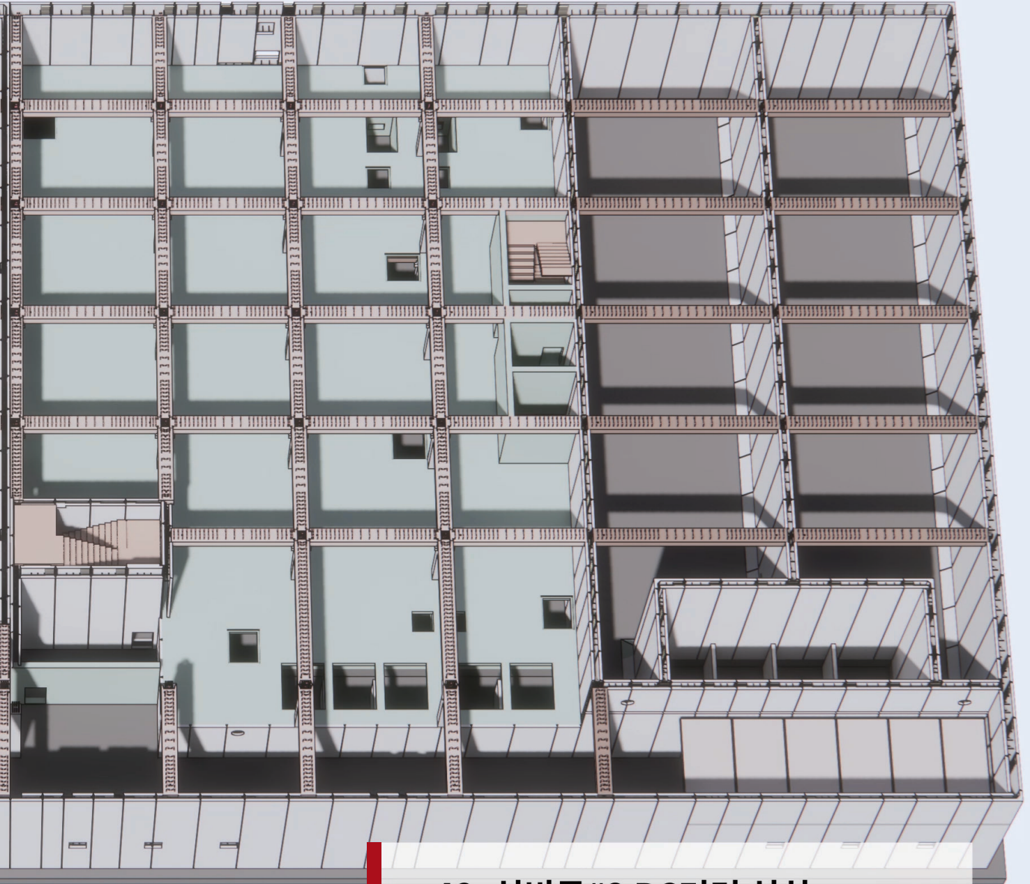
48. 설비동#2 PC거더 설치
