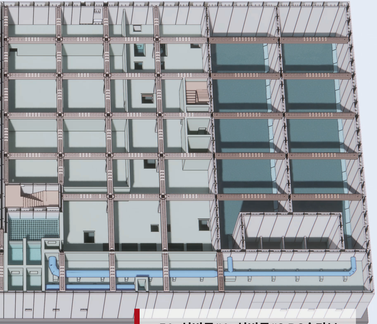
51. 설비동#1, 설비동#2 PC슬라브
